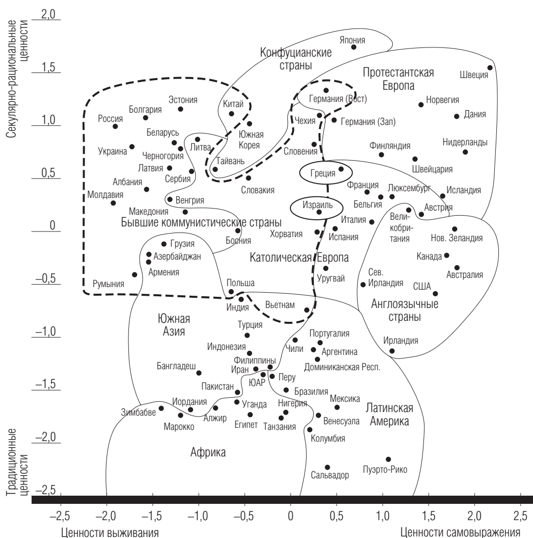
Рисунок 2.4. КУЛЬТУРНАЯ КАРТА МИРА В 2000 ГОДУ
